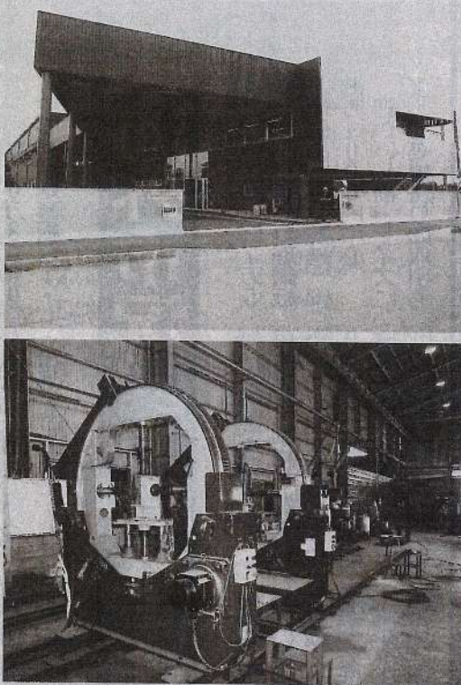
①事務所棟と第5工場(奥)と②新規導入したロボット溶接機
